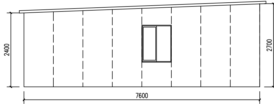
70m 2 Left 1:50
