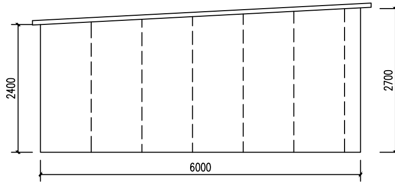
60m 2 Left 1:50
